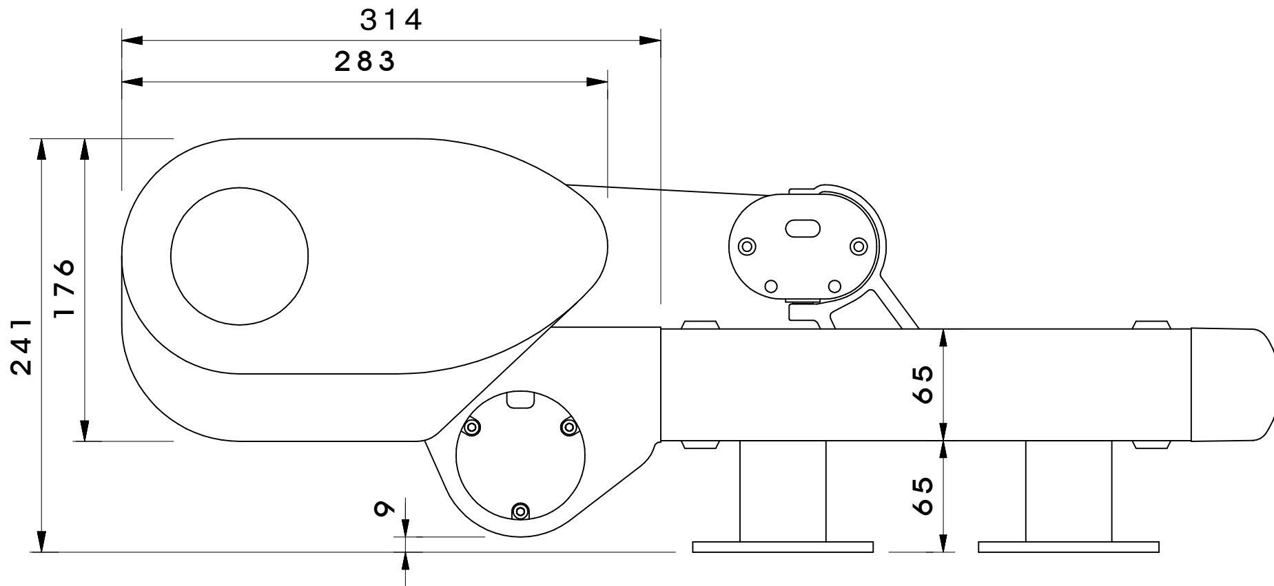
VARISOL W450 Seitenansicht
